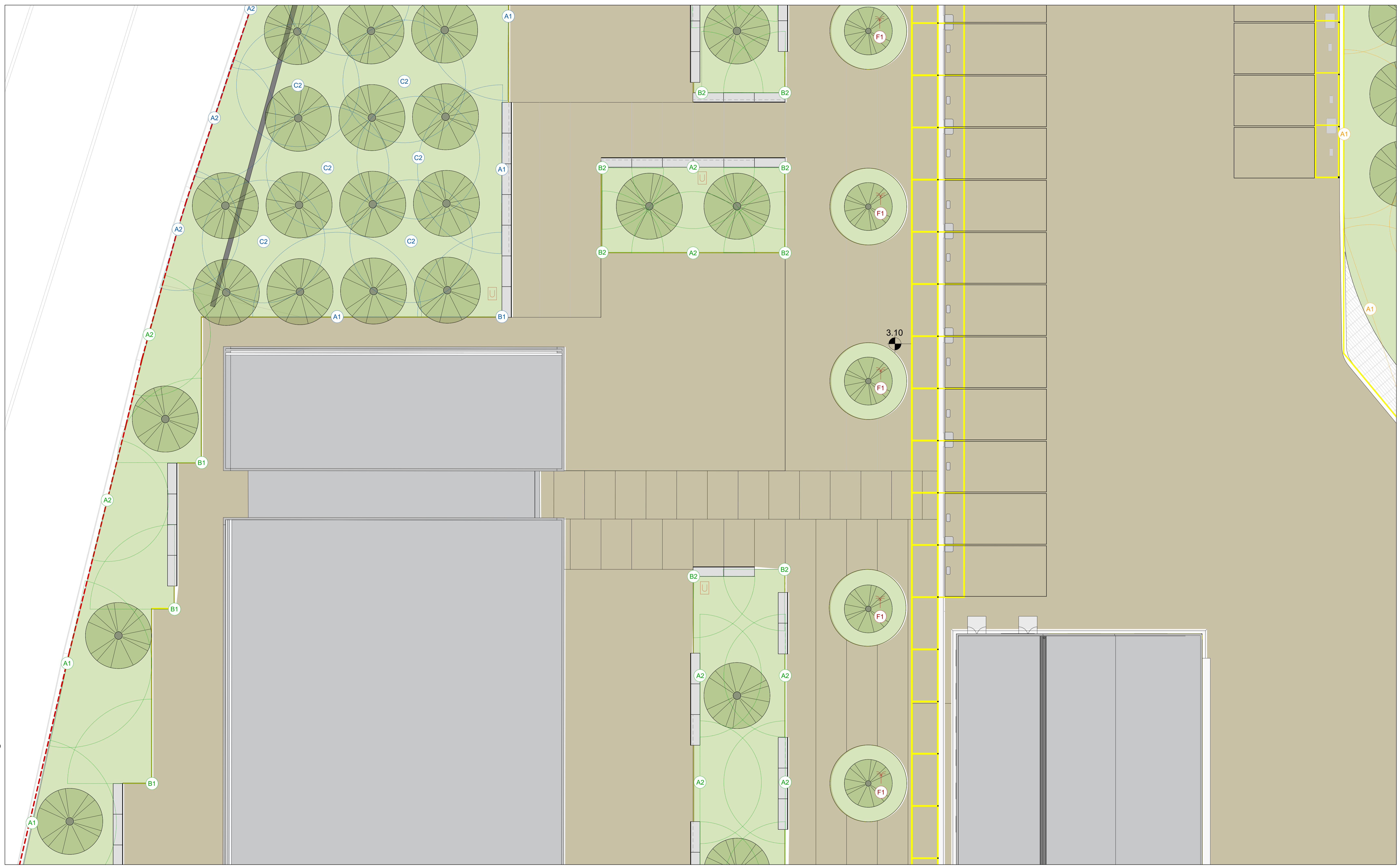
Stralcio planimetrico - scala 1:100
